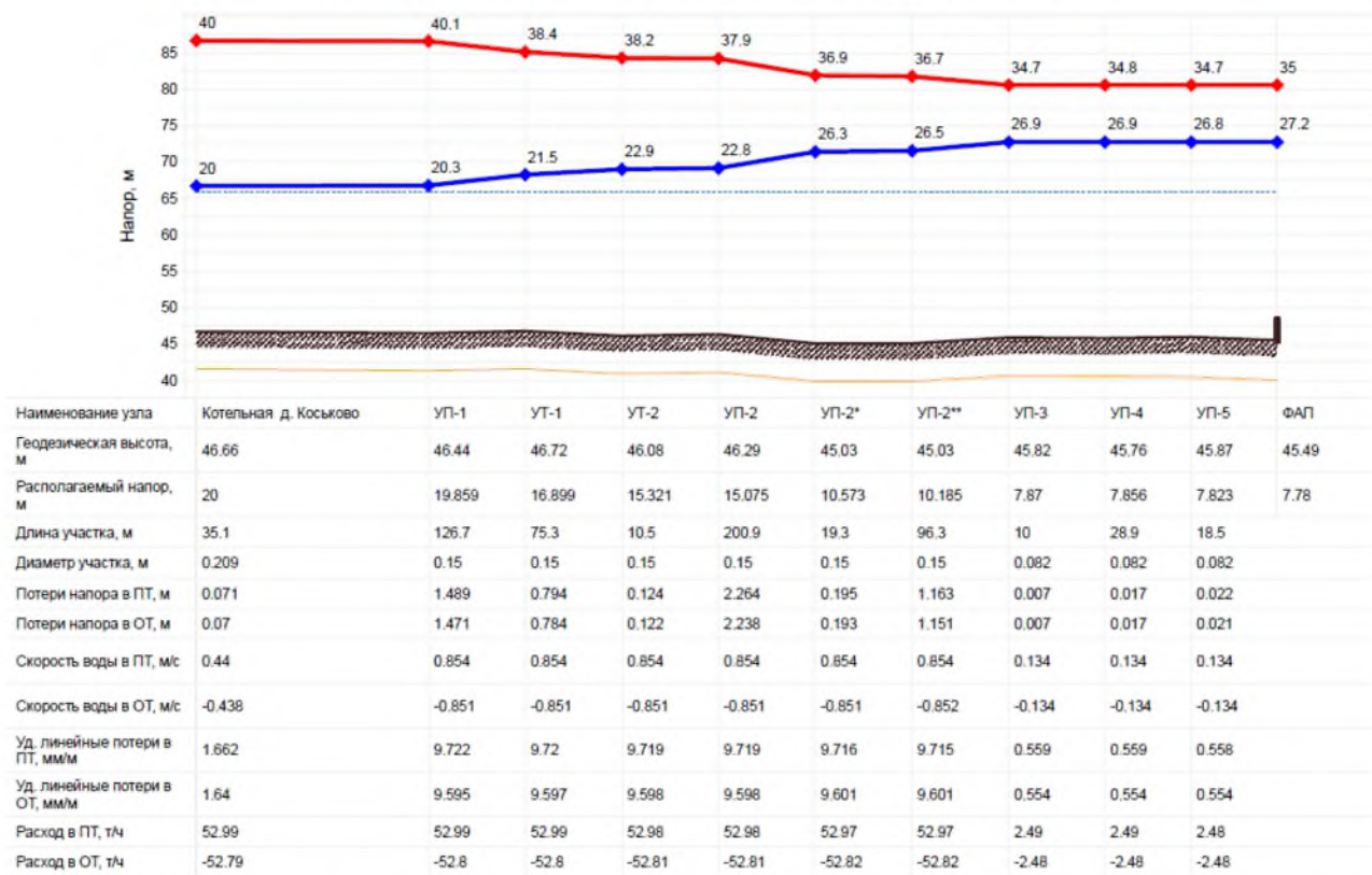
Рисунок 1.3.2 – Пьезометрический график тепловой сети д. Косьюково
