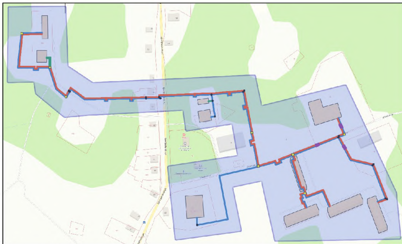
Рисунок 1.4.1 – Зона действия централизованного теплоснабжения котельной в д. Коськово
