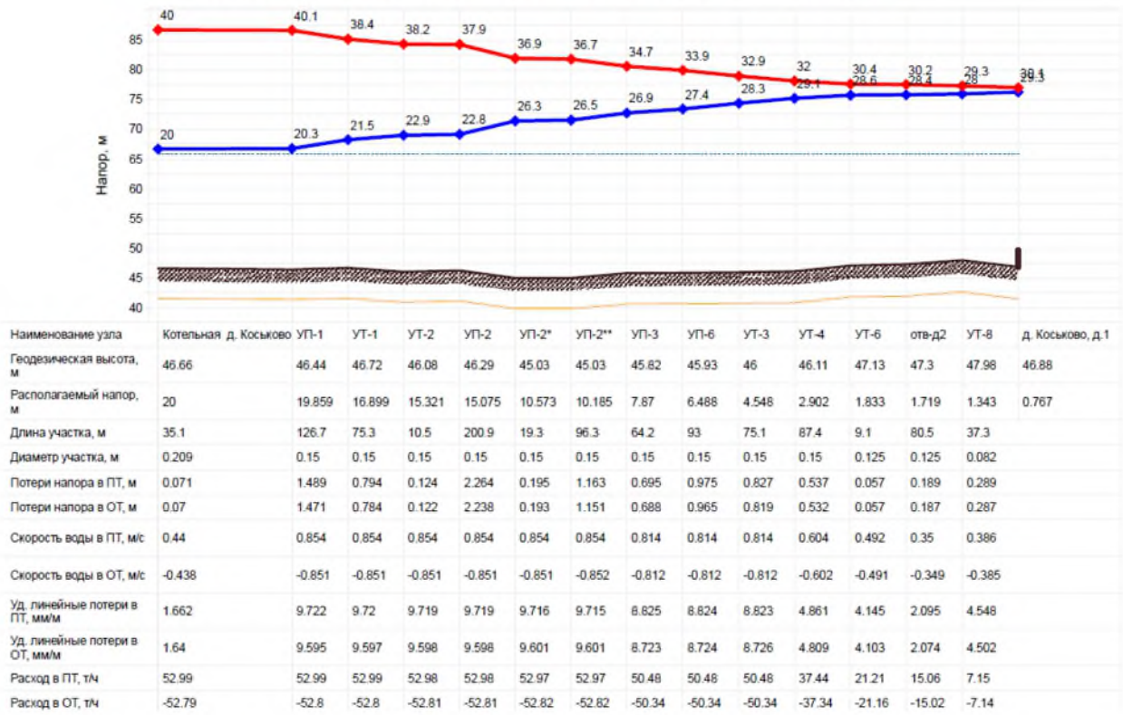
Рисунок 1.3.1 – Пьезометрический график тепловой сети д. Косьюково
