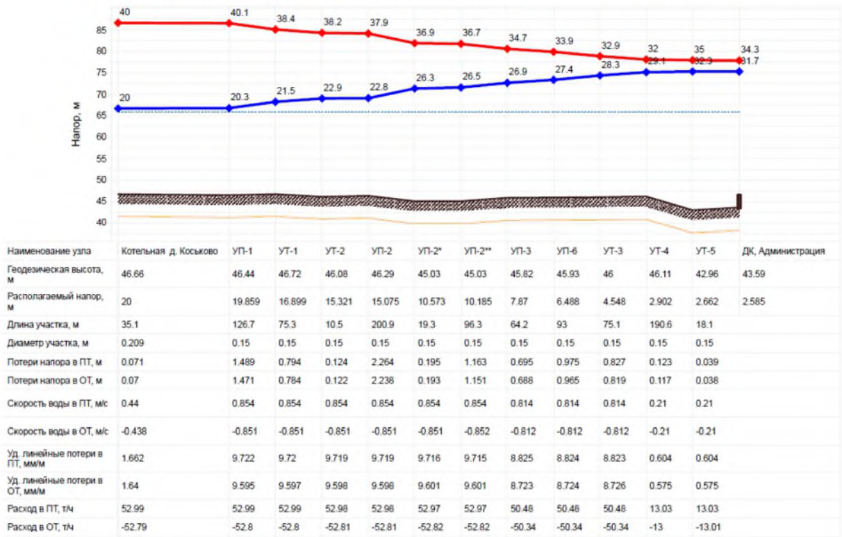
Пьезометрический график от «Котельная д. Коськово» до «ДК, Администрация»
